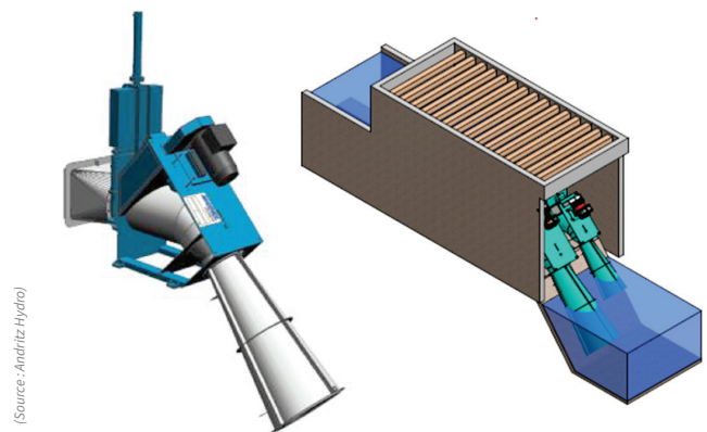
➤ Schéma d'un groupe Andritz Hydro Mini Grid Série intégrant une turbine Kaplan simple réglage
